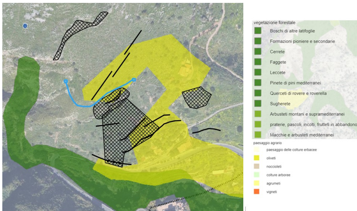
Figura 9: Carta delle componenti del paesaggio. Cerchiato in rosso le pareti sovrastanti Taormina lato mare
