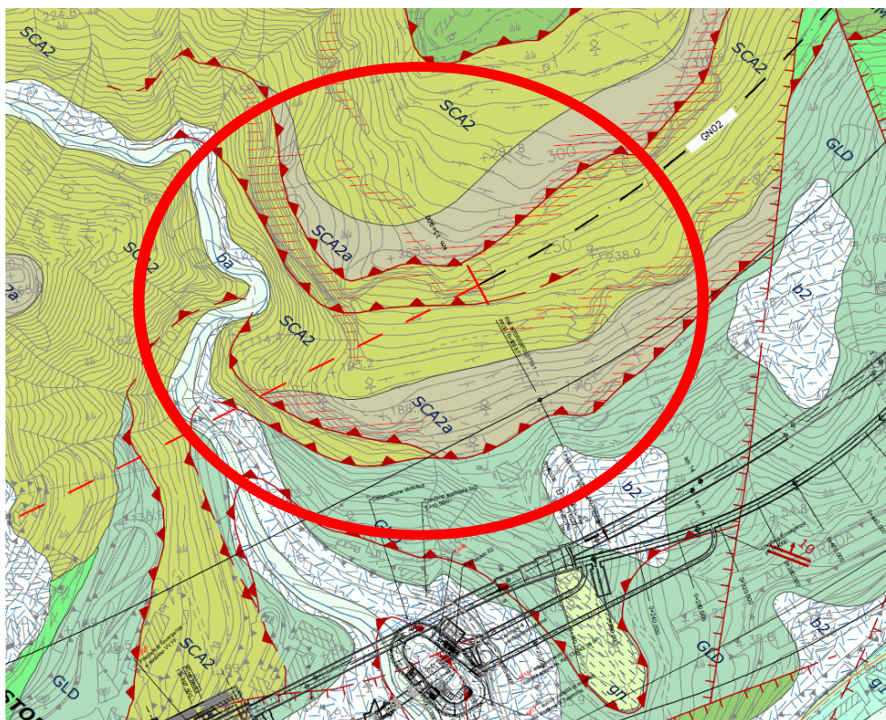
Figura 7: Carta geologica. Cerchiato in rosso le pareti sovrastanti Taormina lato mare
